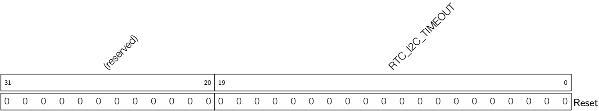
Register 30.11. RTC_I2C_TIMEOUT_REG (0x00c)
